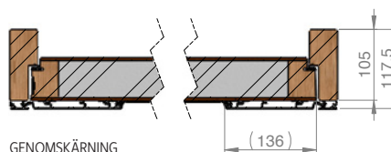
GENOMSKÄRNING
